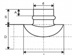
Рис.1 Врезка круглая
