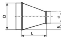
Рис.3 Переход
