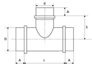
Рис.2 Тройник
